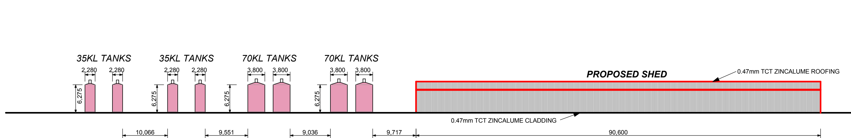
ELEVATION C - C
