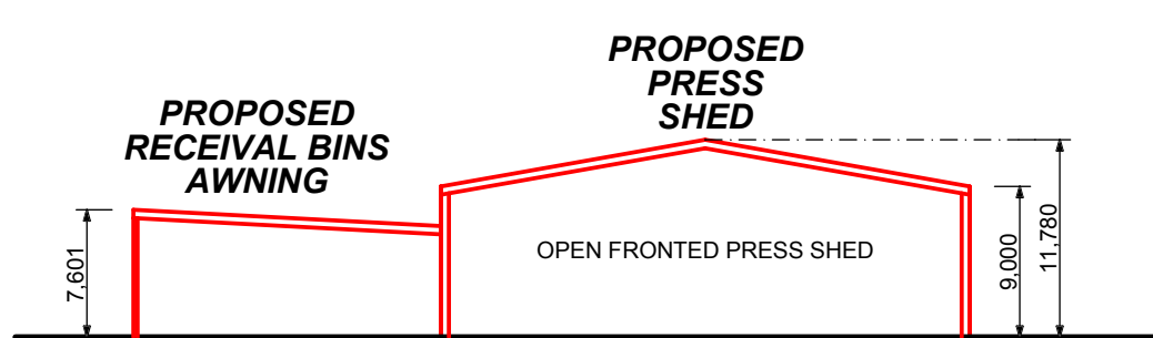
ELEVATION I - I
