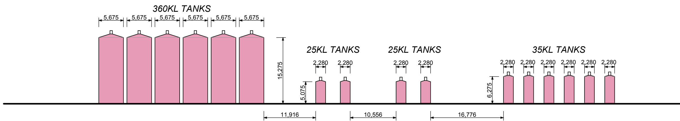
ELEVATION F - F
