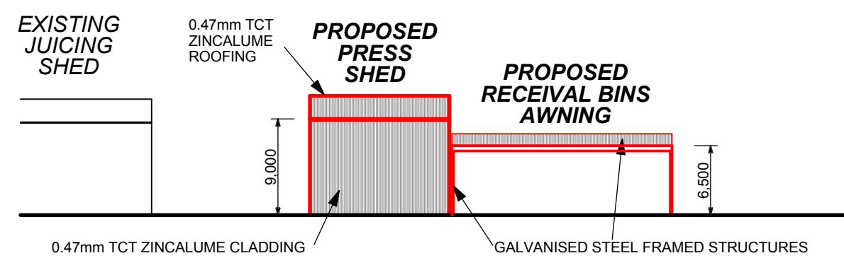
ELEVATION G - G
